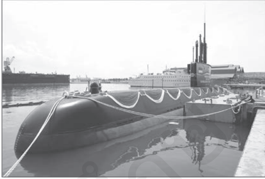
เรือดำน้ำดีเซลไฟฟ้าชั้นซานโบโก (Chang Bogo) ลำที่สาม ชื่อเรืออูลูกโร (KRI Alugoro, 405) ต่อจากคู่อเรือเมืองสุราบายา ประเทศอินโดนีเซีย ประจำปี พ.ศ.๒๕๖๒ ระวังขับน้ำหนัก ๑,๔๐๐ ตัน ยาว ๖๑.๓ เมตร อวูธตอริบีโดชนิด ๘ ท่อยิง (ขนาด ๕๓๓ มิลลิเมตร หรือ ๒๑ นิ้ว แบบ Black Shark)
