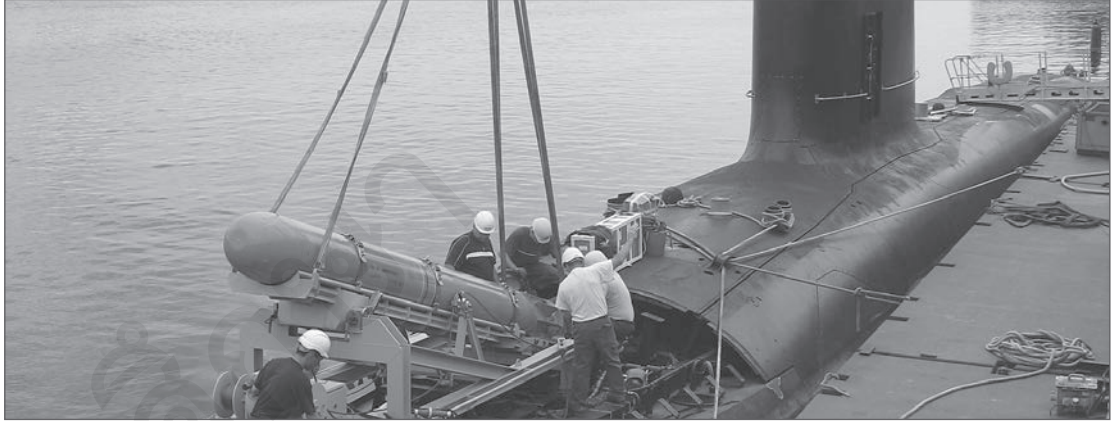
จรวดนำวิถีต่อต้านเรือผิวน้ำแบบเอ็กโซเซต (SM.39 Exocet) กำลังบรรจุลงเรือดำน้ำดีเซลไฟฟ้าชั้นสกอร์ปิเน (Scorpene) ลูกจรวดหนัก ๖๕๕ กิโลกรัม หัวรบหนัก ๑๖๕ กิโลกรัม ความเร็ว ๑,๑๑๓ กิโลเมตรต่อชั่วโมง และระยะยิง ๕๐ กิโลเมตร
