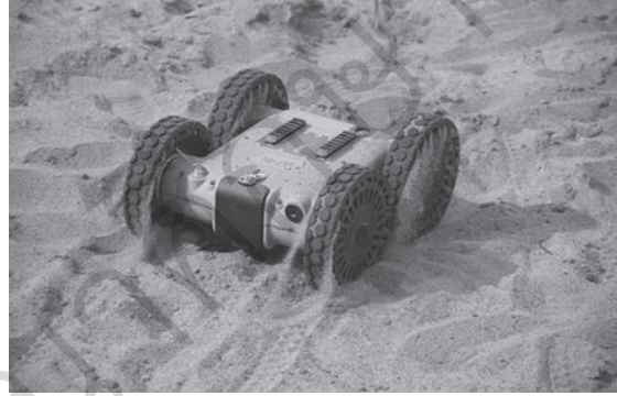
รูปที่ ๓ ต้นแบบหุ่นยนต์ขนาดเล็กแบบพกพา (หนูนา)
