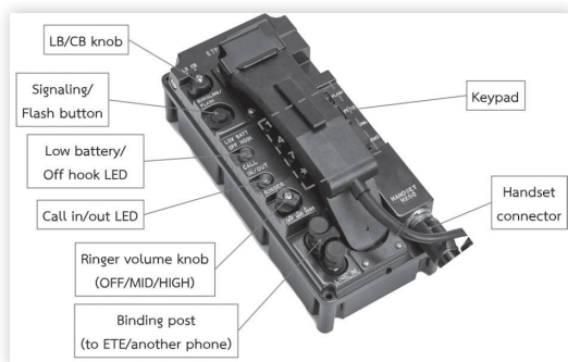
รูป เครื่องโทรศัพท์ ETP-1 (รายละเอียดตัวเครื่อง)
