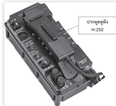
รูป เครื่องโทรศัพท์ ETP-1 (ปากพูดหูฟัง H-250)
