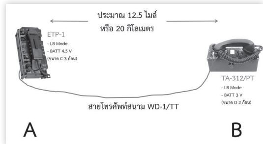
รูป การต่อใช้งานเครื่องโทรศัพท์ ETP-1 และเครื่อง โทรศัพท์ สนามแบบ TA-312/PT
