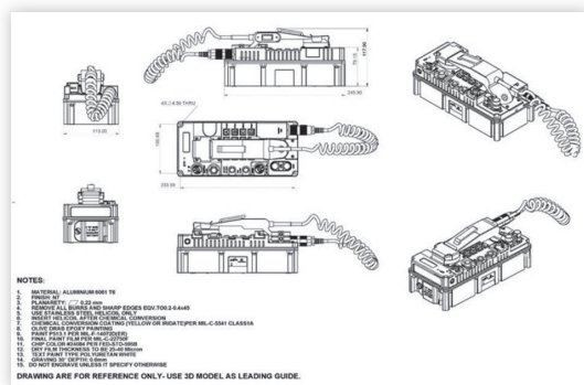
รูป ภาพร่างเครื่องโทรศัพท์ ETP-1 (Out Line)
