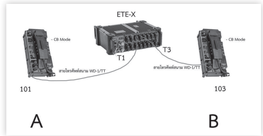
รูป การเชื่อมต่อเครื่องโทรศัพท์ กับเครื่องสลับสายโทรศัพท์ทางทหาร ETE-X
