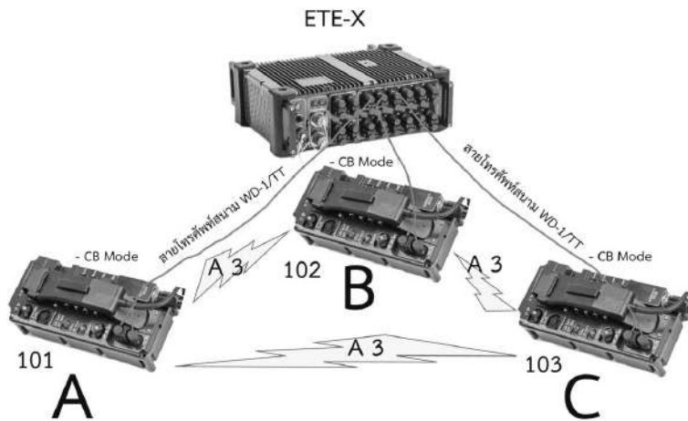
รูป การเชื่อมต่อเครื่องโทรศัพท์ โดยฟังก์ชัน FLASH 3
