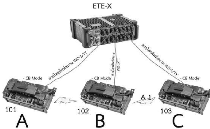
รูป การเชื่อมต่อเครื่องโทรศัพท์ โดยฟังก์ชัน FLASH 1
