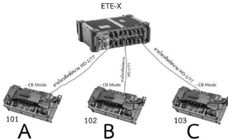
รูป การเชื่อมต่อเครื่องโทรศัพท์ กับเครื่องสลับสายโทรศัพท์ทางทหาร ETE-X
