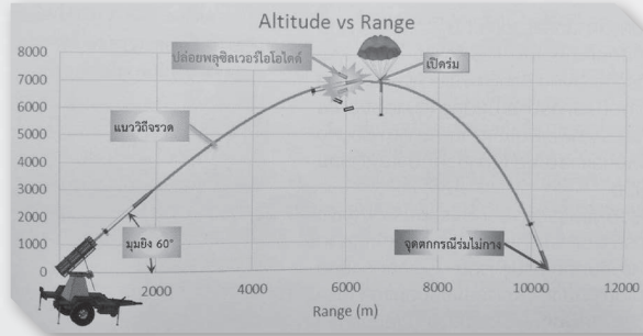
รูปที่ 5 : ลักษณะการทำงานของจรวดดัดแปรสภาพอากาศ
