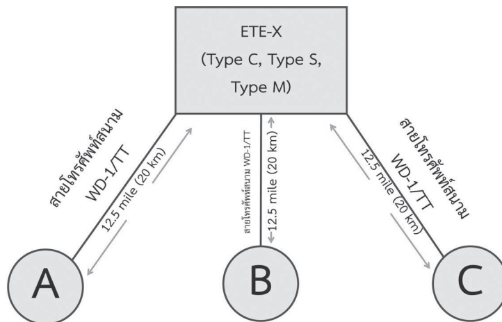
รูป การเชื่อมต่อเครื่องโทรศัพท์ กับเครื่องสลับสายโทรศัพท์ทางทหาร ETE-X
