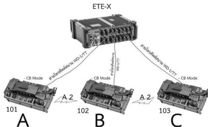
รูป การเชื่อมต่อเครื่องโทรศัพท์ โดยฟังก์ชัน FLASH 2
