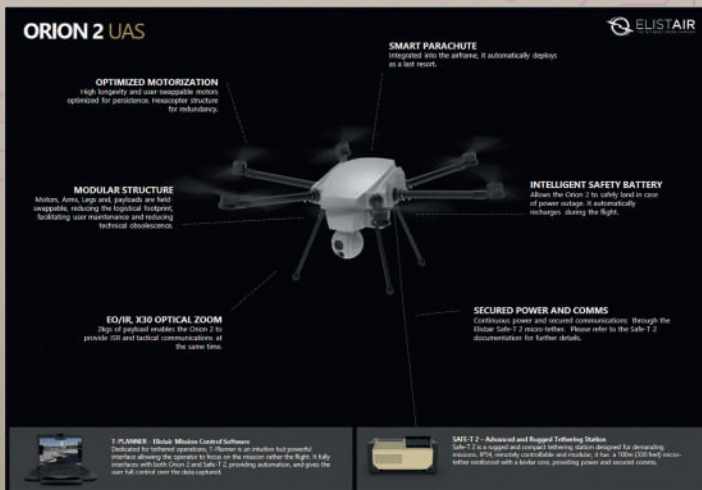
รูปที่ 4 Orion UAS, ผลิตโดย Elistair แพลตฟอร์มนี้มีระดับความสูงในการทำงานถึง 80 เมตร เหมาะสำหรับการติดตั้งระบบโทรคมนาคมที่รวดเร็วในพื้นที่ภัยพิบัติ
