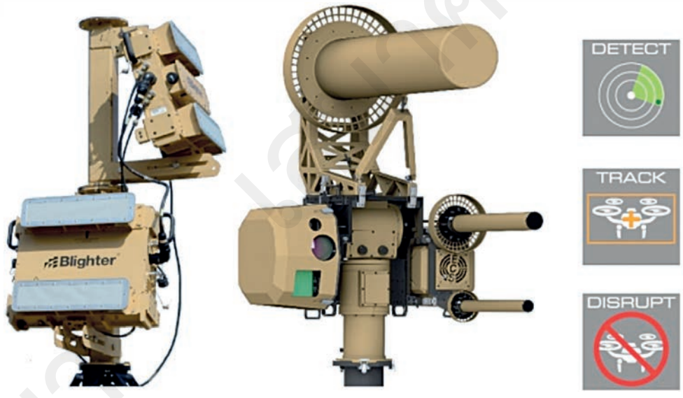
ระบบต่อต้านอากาศยานไร้คนขับ Anti-UAV Defence System ของบริษัท Blighter Surveillance Systems
